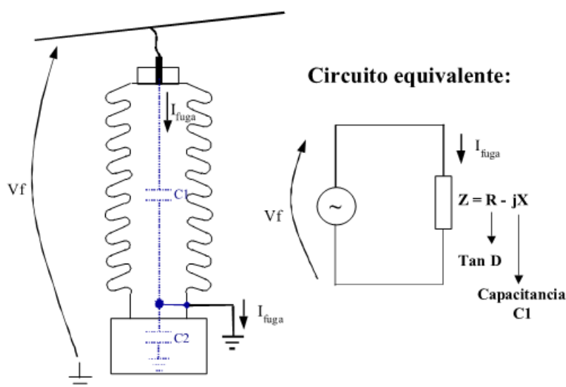
Figura 2 - Circuito equivalente de una bucha condensiva energizada
